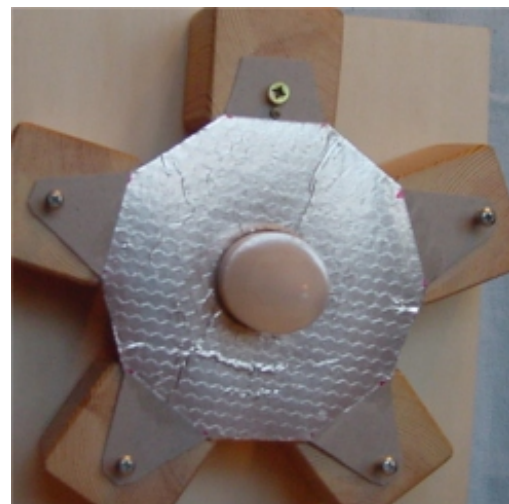
Abbildung: Reflektor mit LED-Farbwechsellampe (230 Volt)
